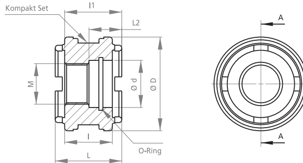
KESİT(SECT.) A-A
